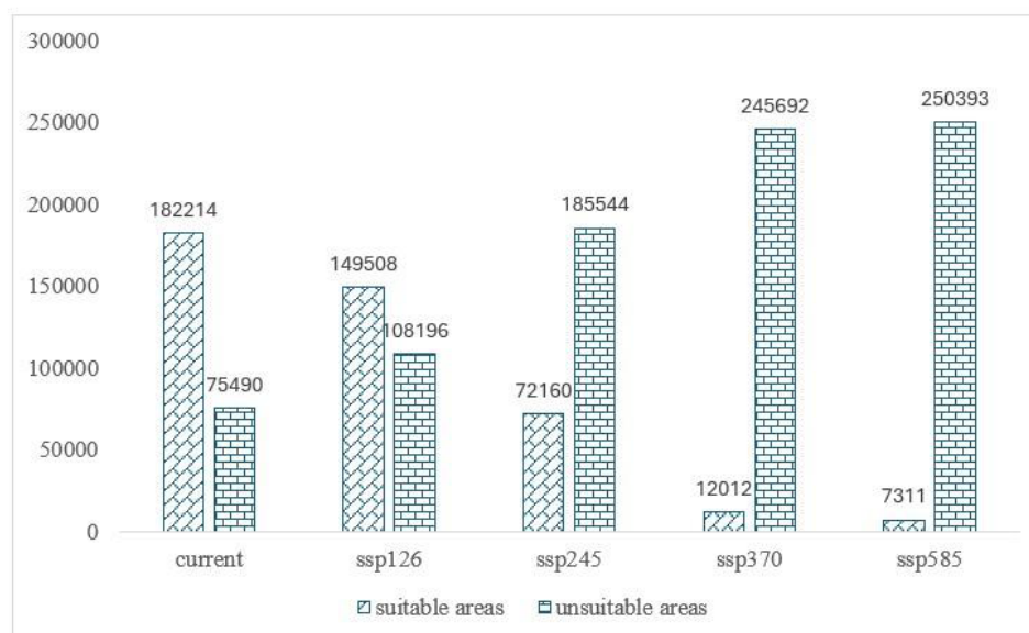
Figure 7. Potential suitable and unsuitable areas of C. monogyna according to present and future climate scenarios Slika 7. Potencijalna prikladna i neprikladna područja za C. monogyna prema sadašnjem i budućem klimatskom scenariju
